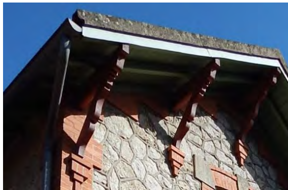
Toiture en saillie de rive avec aisselier
