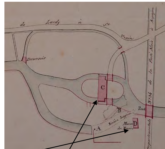
Déplacement du lit de la rivière pour implanter l'actuel moulin - plan de 1836
